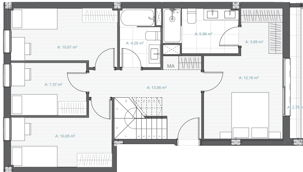
PLANTA TERCERA
