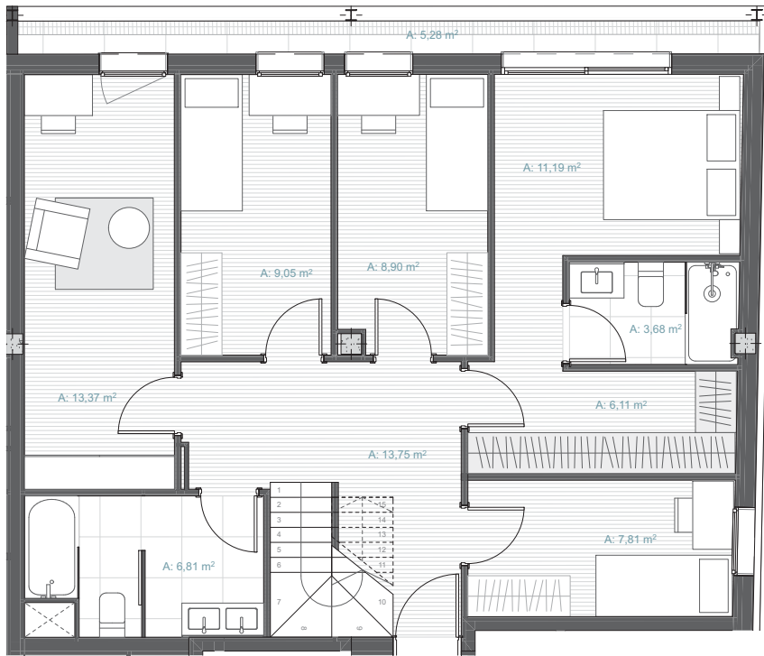
PLANTA TERCERA
