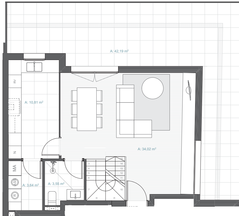
PLANTA SOTACOBERTA
