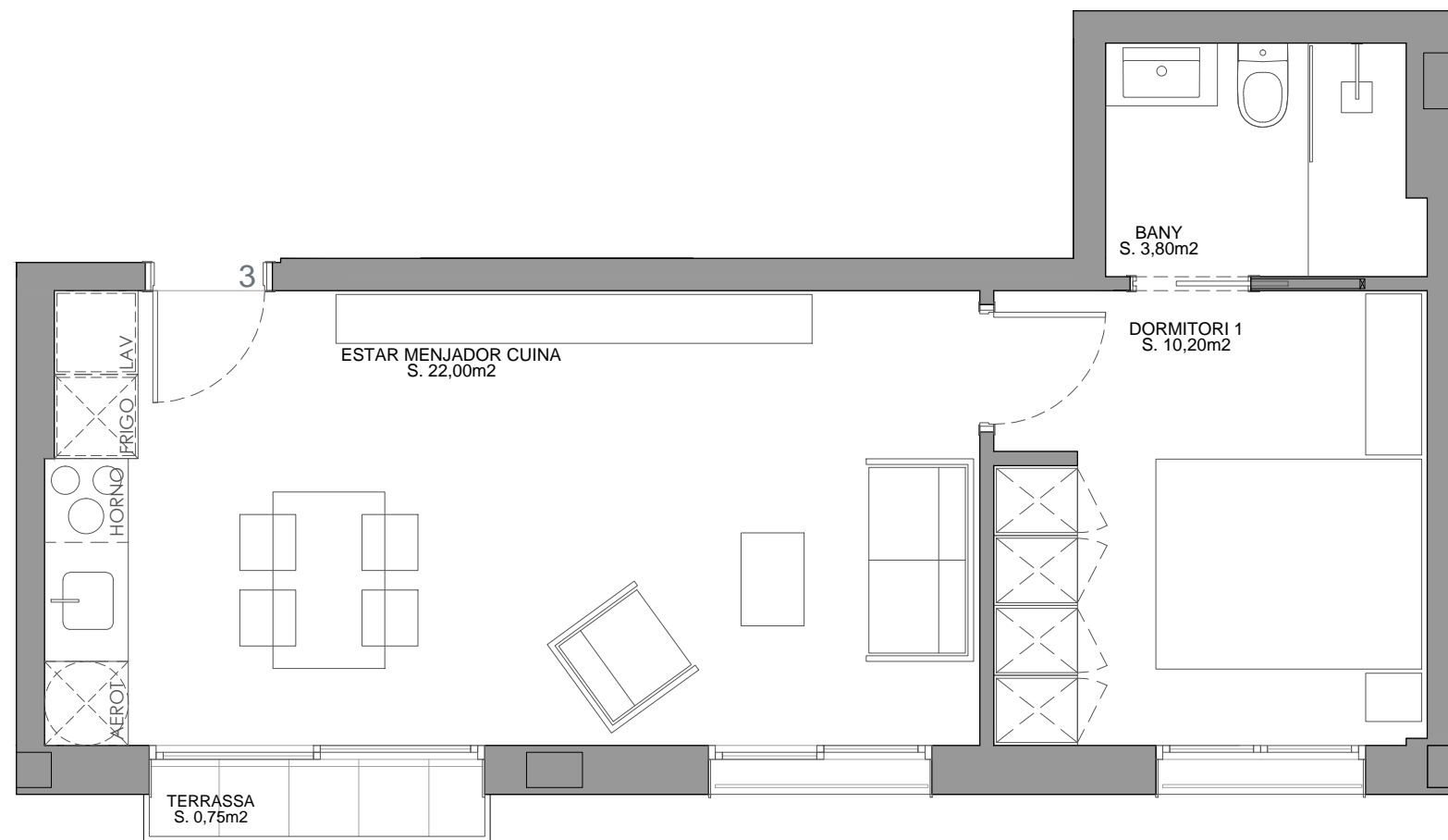
Carrer Dr. Ullés PLANTA SEGONA
