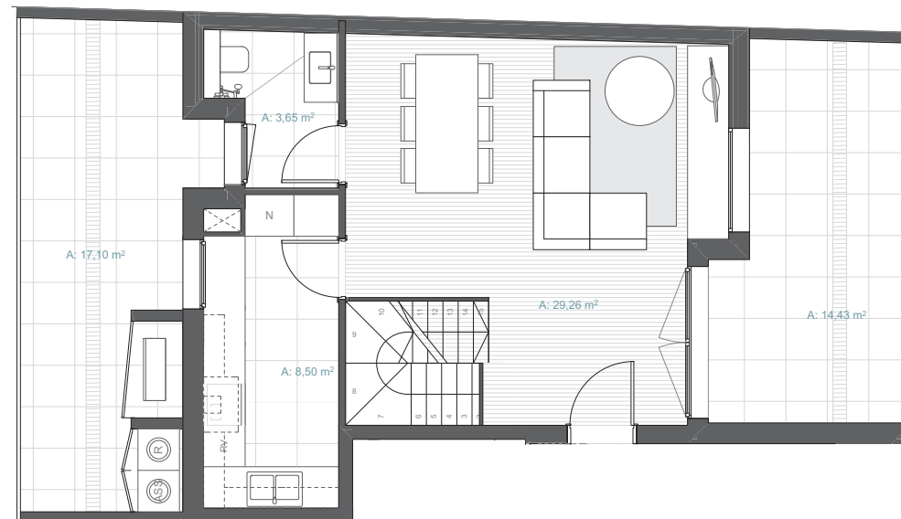
PLANTA SOTACOBERTA
