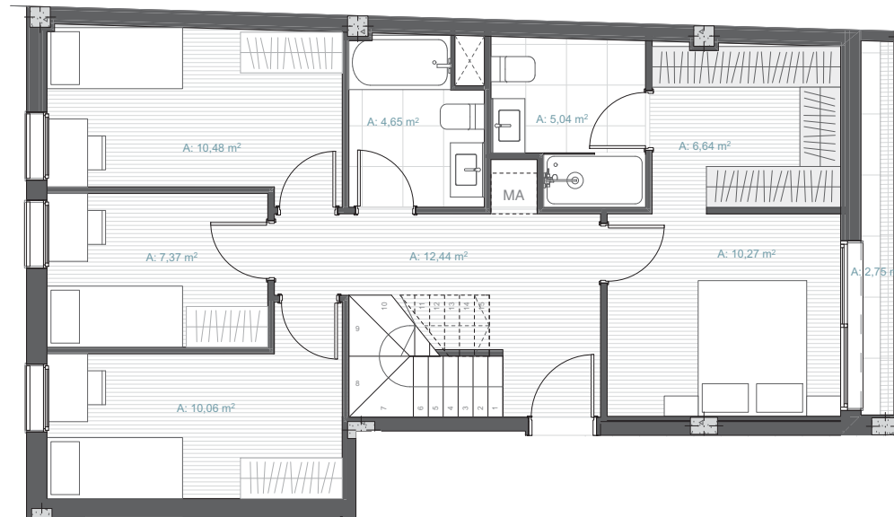
PLANTA TERCERA
