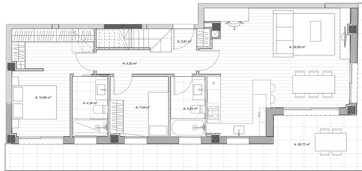
PLANTA CINQUENA
