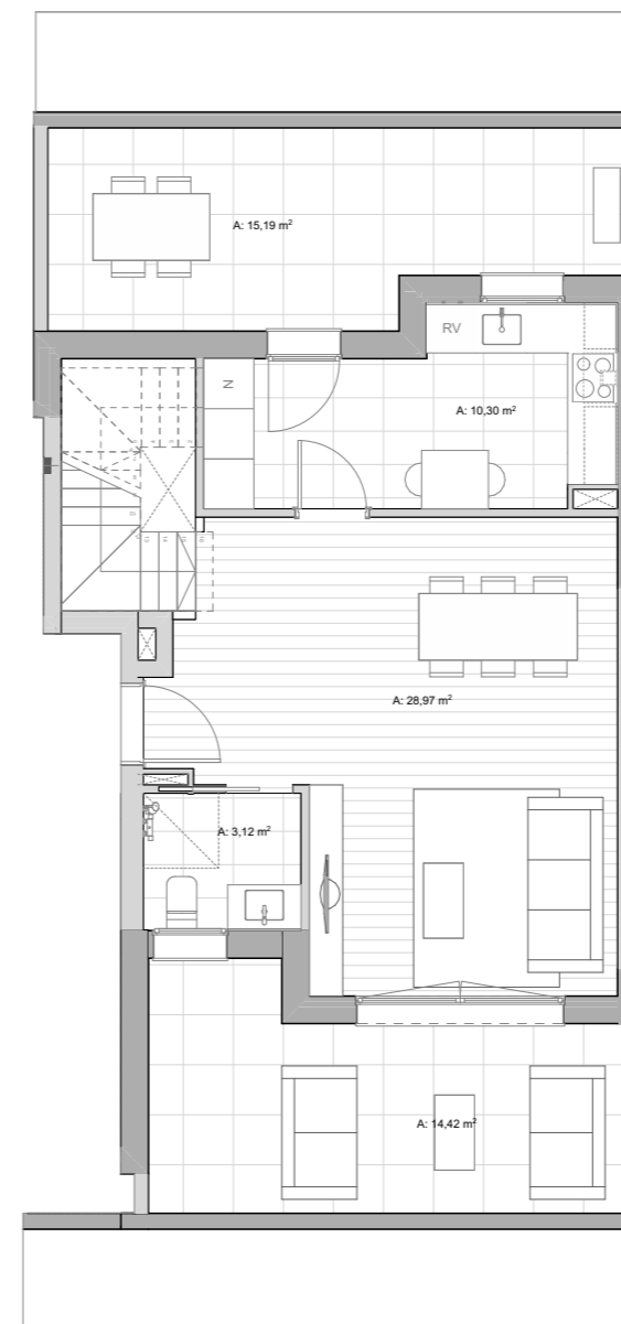
PLANTA SOTACOBERTA
