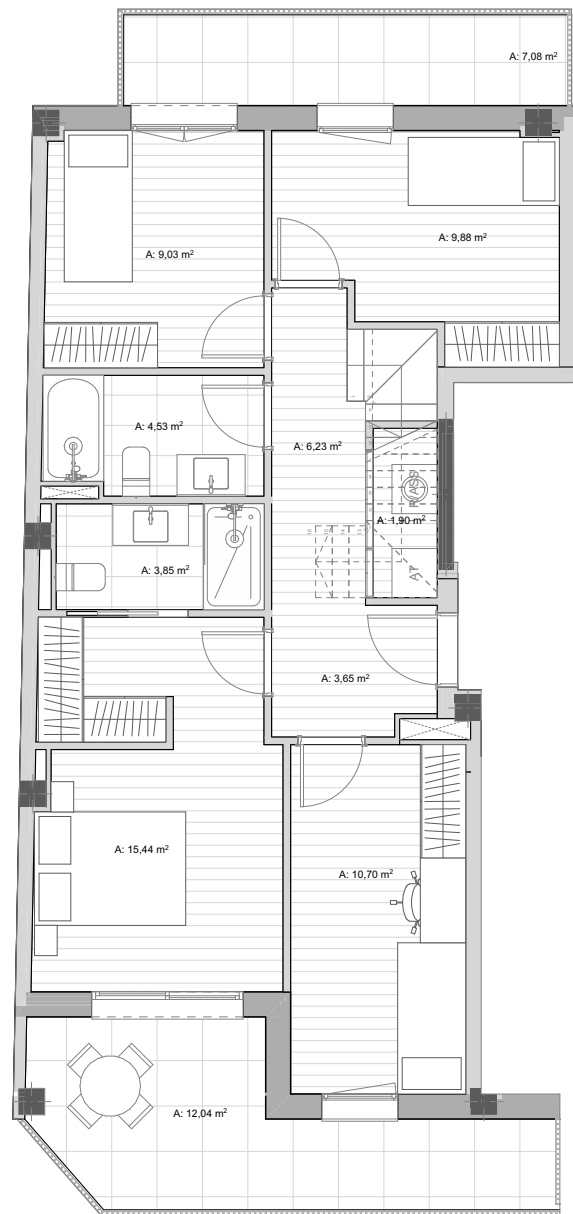
PLANTA CINQUENA
