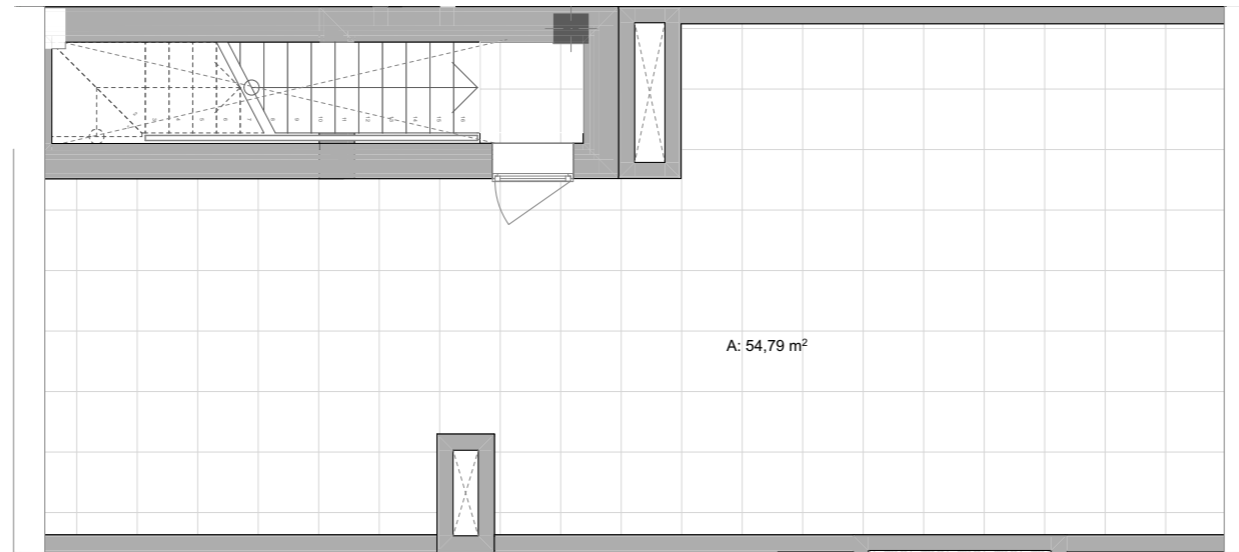
Planta Tercera
